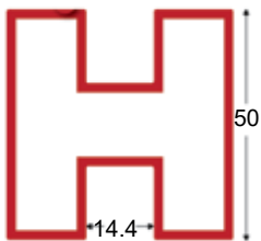
62.052.9157.11 Standprofil 50, 2seitig profil debout 50, double face
