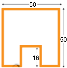
62.052.9152.11 Standprofil 50, 1seitig profil debout 50, unilatéral
